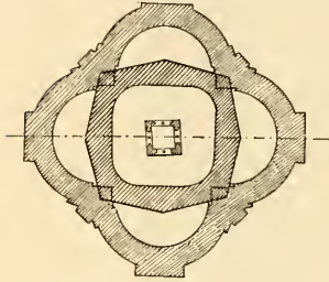
Fig. 375 — Battistero della cattedrale di Biella — Pianta dei due piani e della torricella (sec. X)
